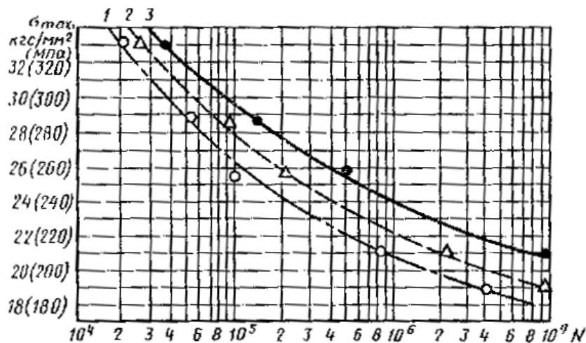
Кривые усталости образцов из сплава марки В95
